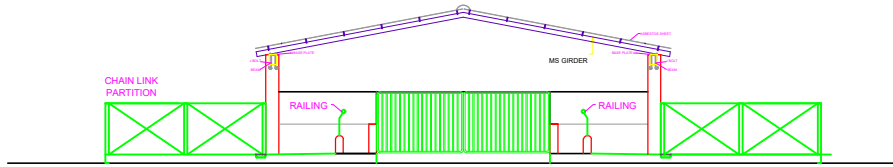
SECTION A-A
